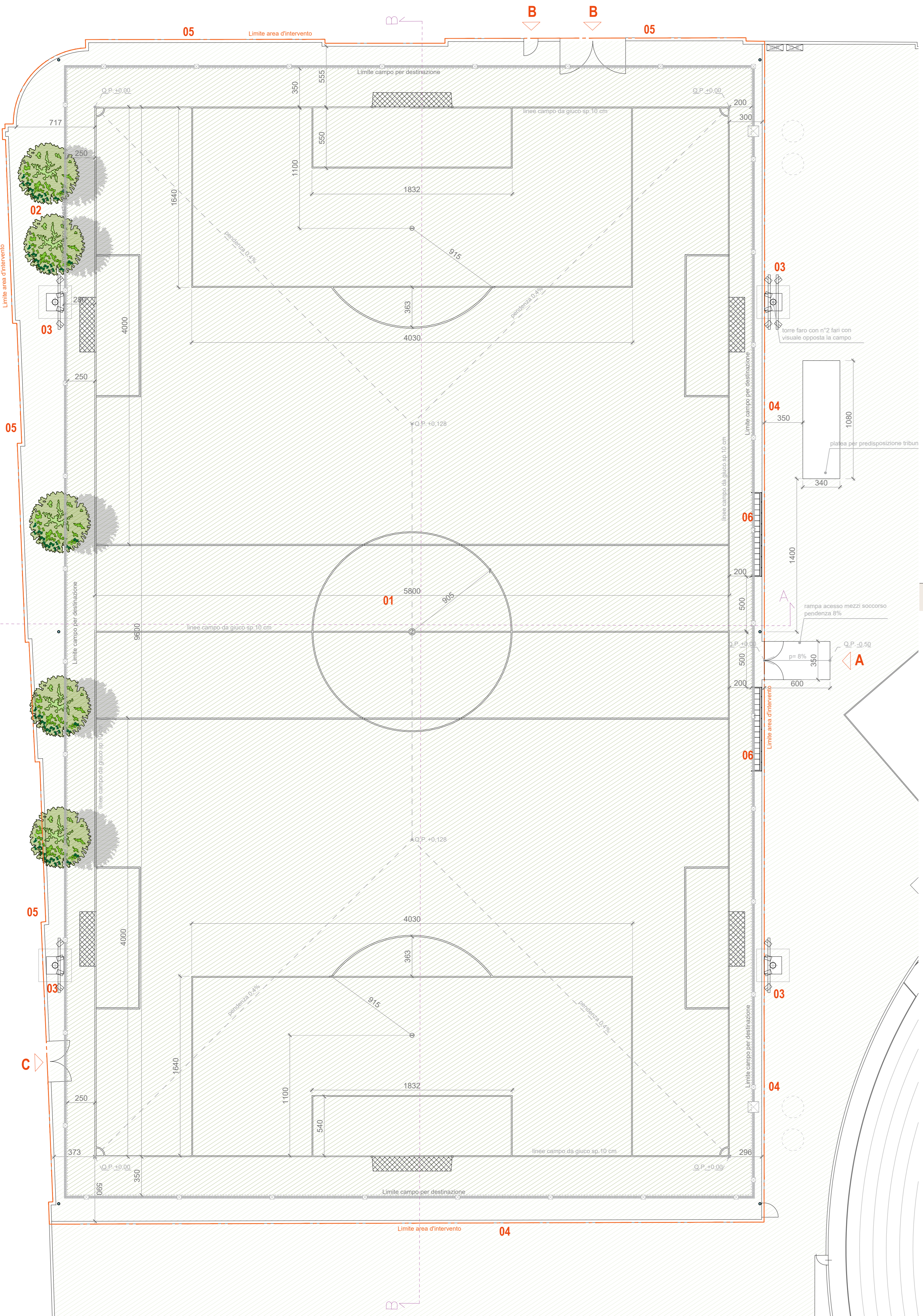
PLANIMETRIA GENERALE STATO DI PROGETTO scala 1:200
