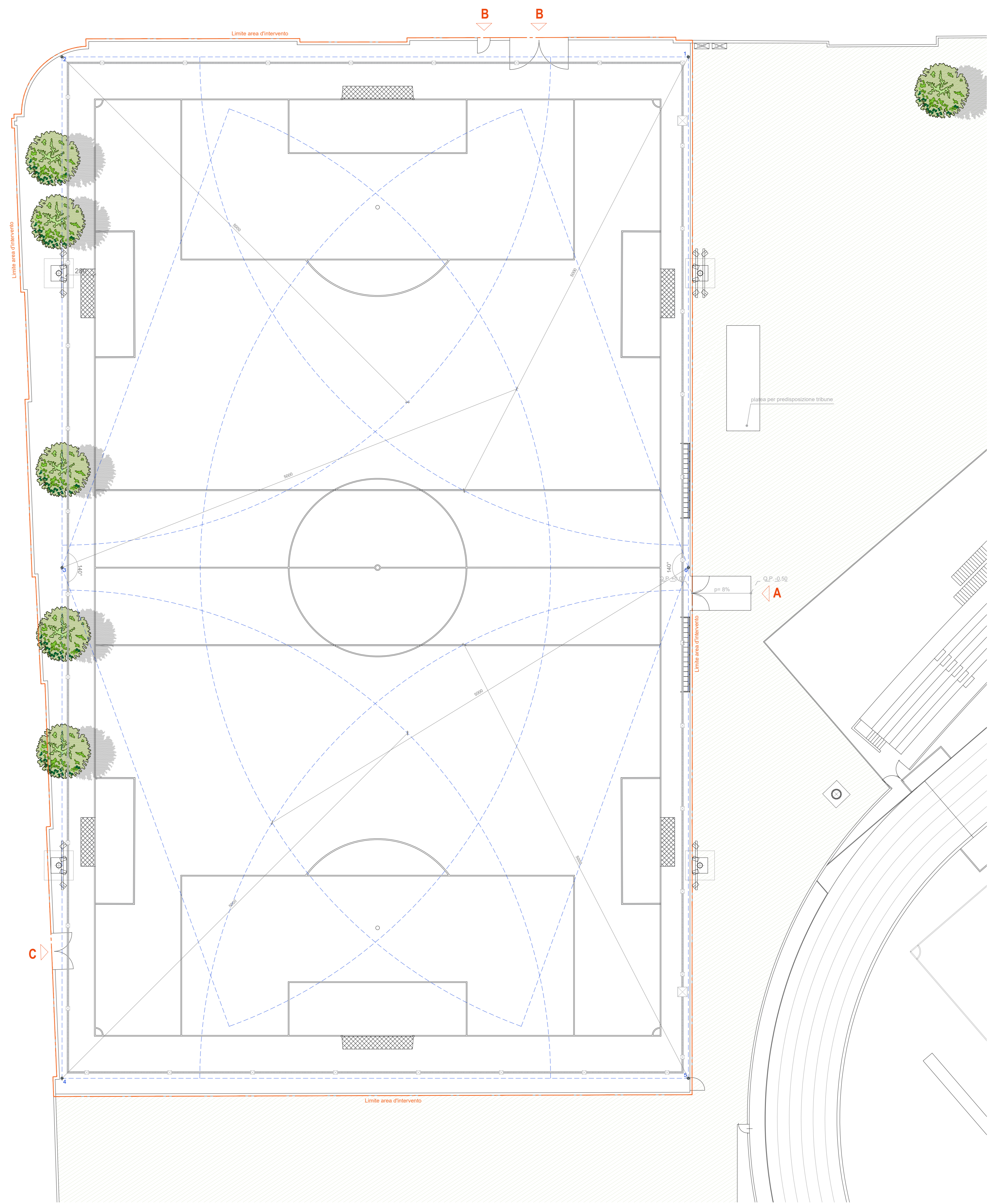
SCHEMA DI IRRIGAZIONE STATO DI PROGETTO scala 1:200
